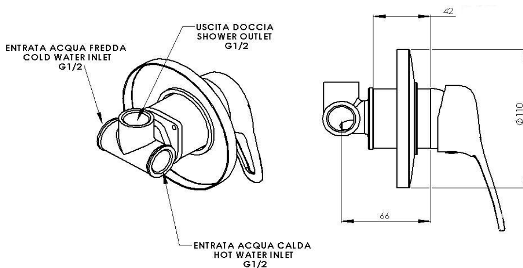
MISCELATORE DA INCASSO X DOCCIA BUILT-IN SHOWER MIXER
